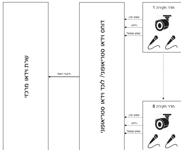
איור 1: ארכיטקטורה לחיבור חדרי חקירה למערכת שרת וידאו מרכזית
